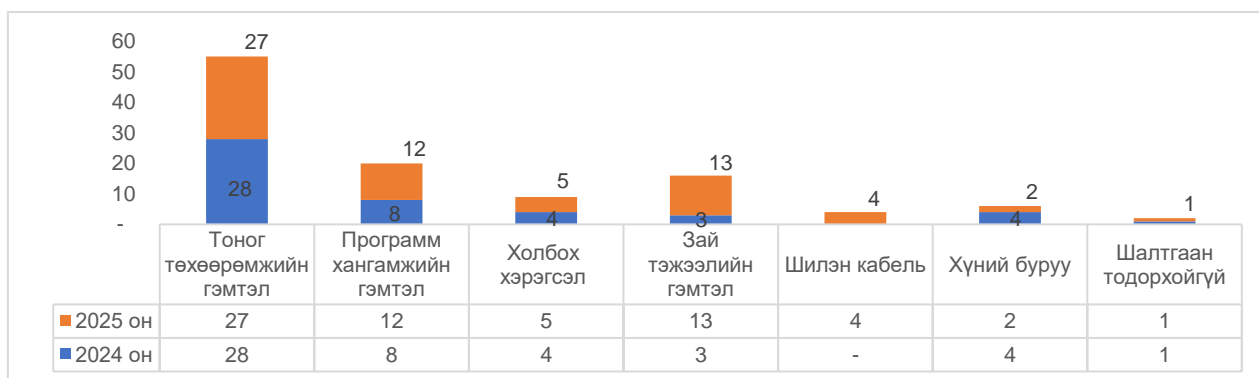
Зураг 13. Өгөгдлийн сүлжээнд гарсан гэмтлийн харьцуулалт
